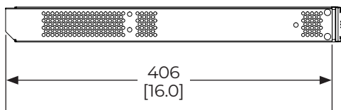
左側視圖
