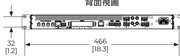
背面視圖
